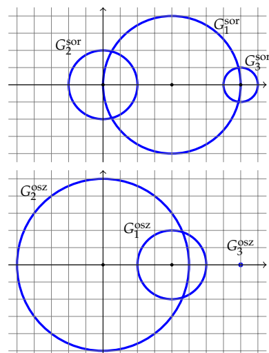
8.3. ábra: Az \mathbf{A} mátrix Gersgorin körei
