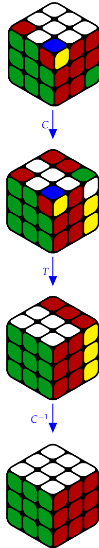
7.17. ábra: A felső kockán látható három csúcskockát kell kicserélni. Először a három csúcsot egy síkba mozgatjuk ( \mathbf{C} transzformáció), majd az előző ábrán látható \mathbf{T} transzformációval kicseréljük őket, végül \mathbf{C} inverzének alkalmazása után minden kocka a helyére kerül. Így a transzformációk egymás utáni elvégzését szorzásnak tekintve a megoldást a \mathbf{C} \mathbf{T} \mathbf{C}^{-1} transzformáció adja.
