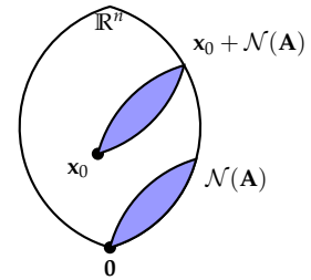
3.8. ábra: Az \mathbf{A} együtthatómátrixú homogén egyenletrendszer megoldása a nulltér, azaz \mathcal{N}(\mathbf{A}) , az inhomogéné e tér egy \mathbf{x}_0 + \mathcal{N}(\mathbf{A}) eltolja, ahol \mathbf{x}_0 az inhomogén egyenletrendszer egy megoldása.
