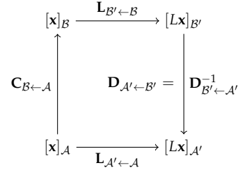
7.18. ábra: Az ábráról leolvasható az \mathbf{L}_{\mathcal{A}' \leftarrow \mathcal{A}} = \mathbf{D}_{\mathcal{A}' \leftarrow \mathcal{B}'}\mathbf{L}_{\mathcal{B}' \leftarrow \mathcal{B}}\mathbf{C}_{\mathcal{B} \leftarrow \mathcal{A}} , illetve az \mathbf{L}_{\mathcal{A}' \leftarrow \mathcal{A}} = \mathbf{D}_{\mathcal{B}' \leftarrow \mathcal{A}'}^{-1}\mathbf{L}_{\mathcal{B}' \leftarrow \mathcal{B}}\mathbf{C}_{\mathcal{B} \leftarrow \mathcal{A}} összefüggés. Ehhez az [\mathbf{x}]_{\mathcal{A}} -ból az [L\mathbf{x}]_{\mathcal{A}'} -be vezető két utat kell bejárunk, és közben a megfelelő mátrixokat összeszorozunk.
