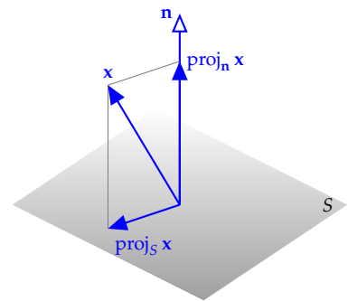
7.11. ábra: Vektor vetülete egy síkra
