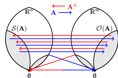
7.20. ábra: Az \mathbf{A} mátrix sortere és oszloptere közti kölcsönösen egyértelmű leképezés a pszeudoinverz fogalmának alapja.
