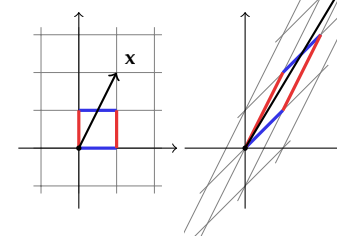
7.5. ábra: Az \mathbf{A} = \begin{bmatrix} 1 & 1 \\ 1 & 2 \end{bmatrix} mátrix hatása az egységnégyzetrácson, és az \mathbf{x} = (1,2) vektoron. Az \mathbf{Ax} vektor végpontja a parallelogrammarácson 1 lépés az x -tengely képének irányába, és 2 lépés az y -tengely képének irányába.
