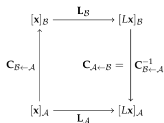
7.15. ábra: Ezt az ábrát az előzőből egyetlen nyíl és felírata megváltoztatásával kaptuk. Erről közvetlenül leolvasható az L_{\mathcal{A}} = C_{\mathcal{A} \leftarrow \mathcal{B}}L_{\mathcal{B}}C_{\mathcal{B} \leftarrow \mathcal{A}} , illetve az L_{\mathcal{A}} = C_{\mathcal{B} \leftarrow \mathcal{A}}^{-1}L_{\mathcal{B}}C_{\mathcal{B} \leftarrow \mathcal{A}} összefüggés. Ehhez az [x]_{\mathcal{A}} -ból az [Lx]_{\mathcal{A}} -ba vezető két utat kell bejárnunk, és közben a megfelelő mátrixokat összeszoroznunk.
