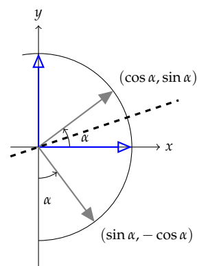
7.12. ábra: Az \mathbf{i} és \mathbf{j} vektorok egy egyenesre való tükörképe
