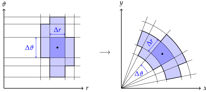
7.26. ábra: A síkbeli polárkoordináta-rendszerre való áttérést megadó leképezés szemléltetése egy téglányokból álló tartomány képének ábrázolásával.
