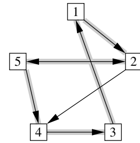
12.1. ábra: Az \mathbf{A} és \mathbf{B} mátrixokhoz rendelt két gráf.
