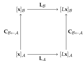
7.14. ábra: A vízszintes nyilak az L transzformáció hatását mutatják. E hatás elérhető az L_{\mathcal{A}} , illetve az L_{\mathcal{B}} mátrixszal való szorzással. A függőleges nyilak a báziscsere irányát mutatják, ami a C_{\mathcal{B} \leftarrow \mathcal{A}} mátrixszal való szorzással valósítható meg. Az ábráról leolvasható a L_{\mathcal{B}}C_{\mathcal{B} \leftarrow \mathcal{A}} = C_{\mathcal{B} \leftarrow \mathcal{A}}L_{\mathcal{A}} összefüggés.
