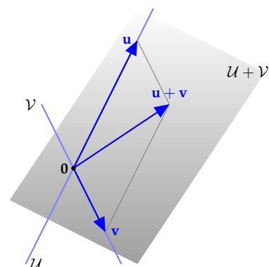
7.19. ábra: \mathcal{U} + \mathcal{V} bármely vektora előáll \mathbf{u} + \mathbf{v} alakban
