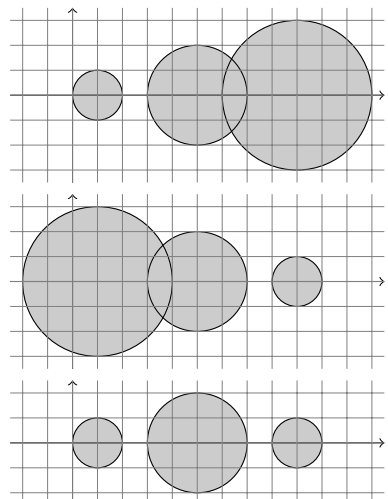
8.5. ábra: A \mathbf{B} mátrix sorösszeg és oszlopösszeg szerinti Gersgorin körei és ezek metszete. Utóbbi mutatja, hogy \mathbf{B} -nek három valós sajátértéke van.
