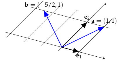
1.41. ábra: Két vektor skaláris szorzata
