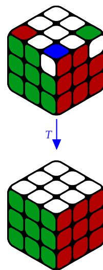
7.16. ábra: A T transzformáció a bűvös kocka egy lapon lévő 3 csúcsát ciklikusan fölcseréli egymással (a jobb felső sarokban lévő a bal sarokba, azt a középsőbe viszi), az összes többi helyben hagyja.
