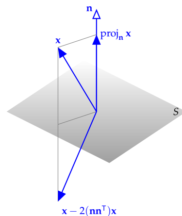
7.13. ábra: Vektor tükörképe egy síkra
